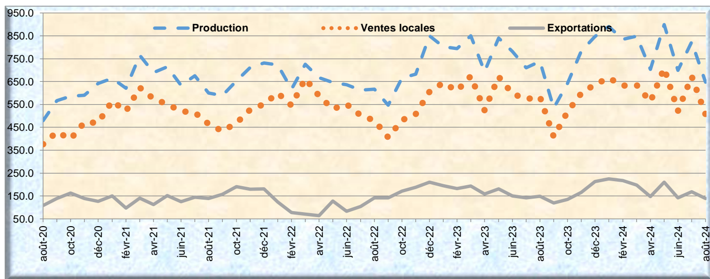
Graphique 5 : Evolution de la production, des ventes locales et des exportations de ciment (en milliers de tonnes)
