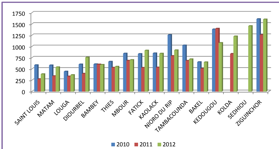
Graphique 9.1 : Cumul de pluies de quelques stations (en mm)
