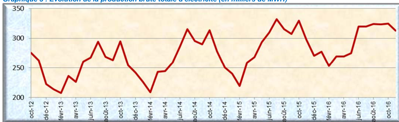
Graphique 3 : Evolution de la production brute totale d'électricité (en milliers de MWH)
