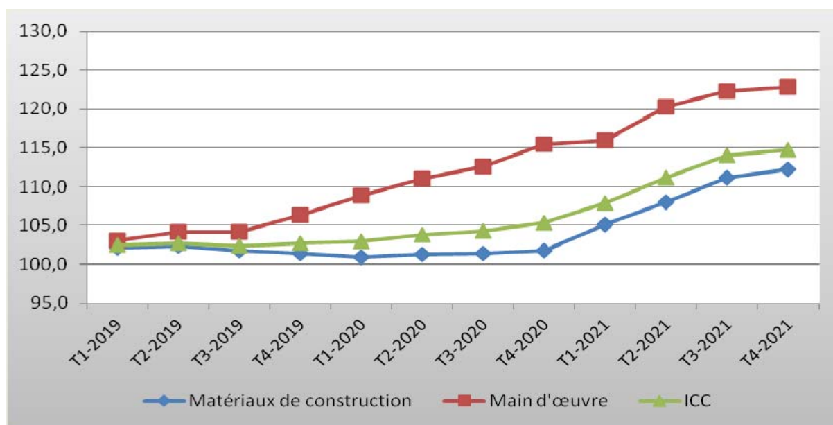
Graphique 10 : Evolutions de l'indice global et des sous indices des coûts de construction
