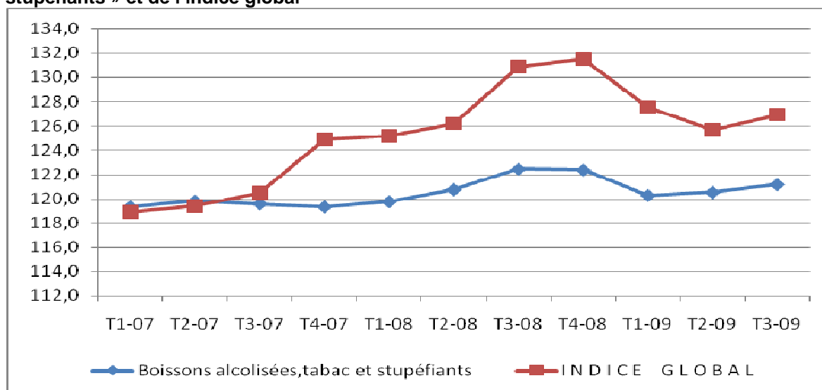
Graphique 10: Evolution trimestrielle de la fonction « boissons alcoolisées, tabacs et stupéfiants » et de l'indice global
