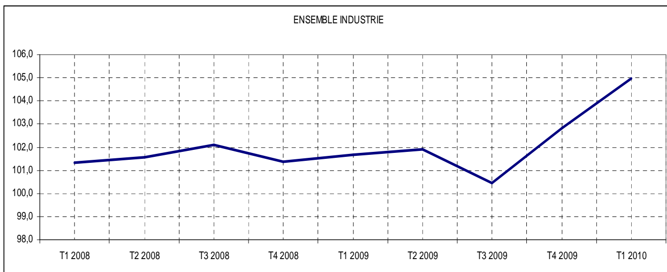
Graphique 1 : Evolution de l'indice d'ensemble des prix à la production industrielle
